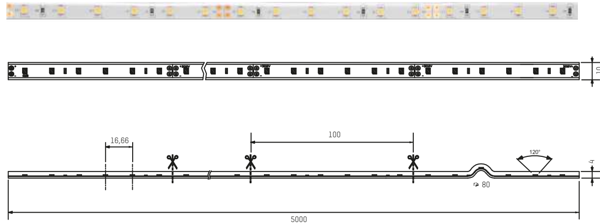
FLEX.light 4,8W ACHTUNG: maximale Länge pro Einspeisepunkt 5m LED/ Attention: Maximum length per feed point 5m
