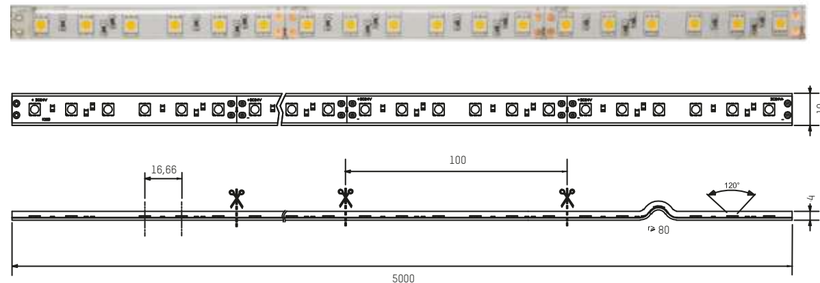
FLEX.light 14,4W ACHTUNG: maximale Länge pro Einspeisepunkt 5m LED/ Attention: Maximum length per feed point 5m
